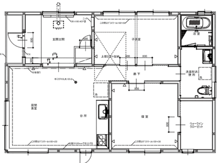
間取り図 A棟
