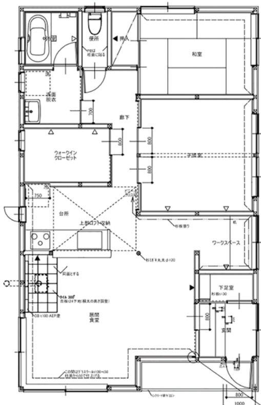
間取り図 B棟
